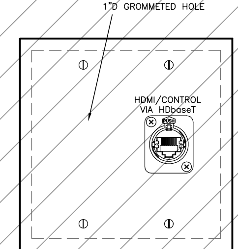
AVP-113 OFFSTAGE VID MON; 2-GANG; FLUSH-MOUNT
