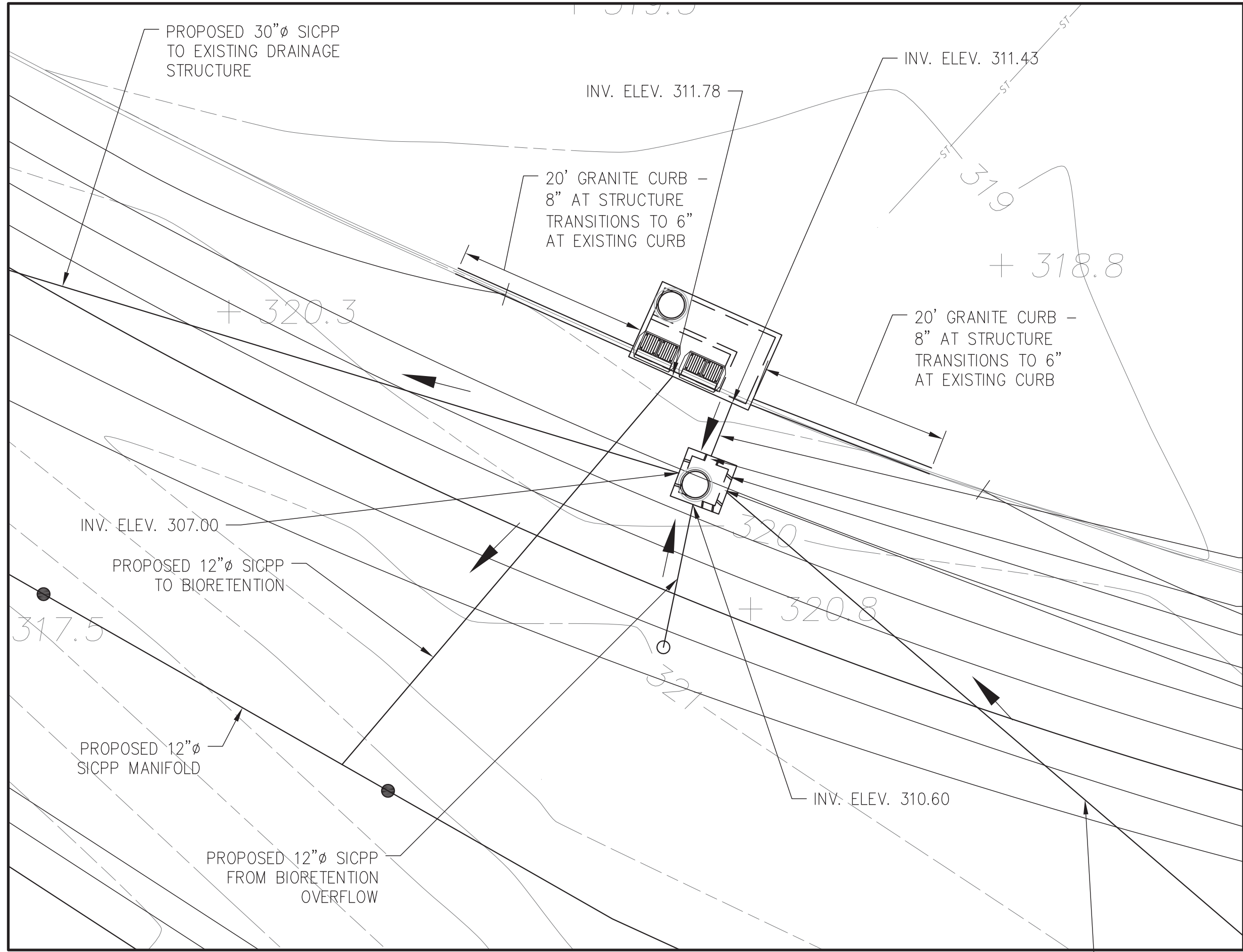
S3 PLAN SCALE: 1" = 10'-0"
