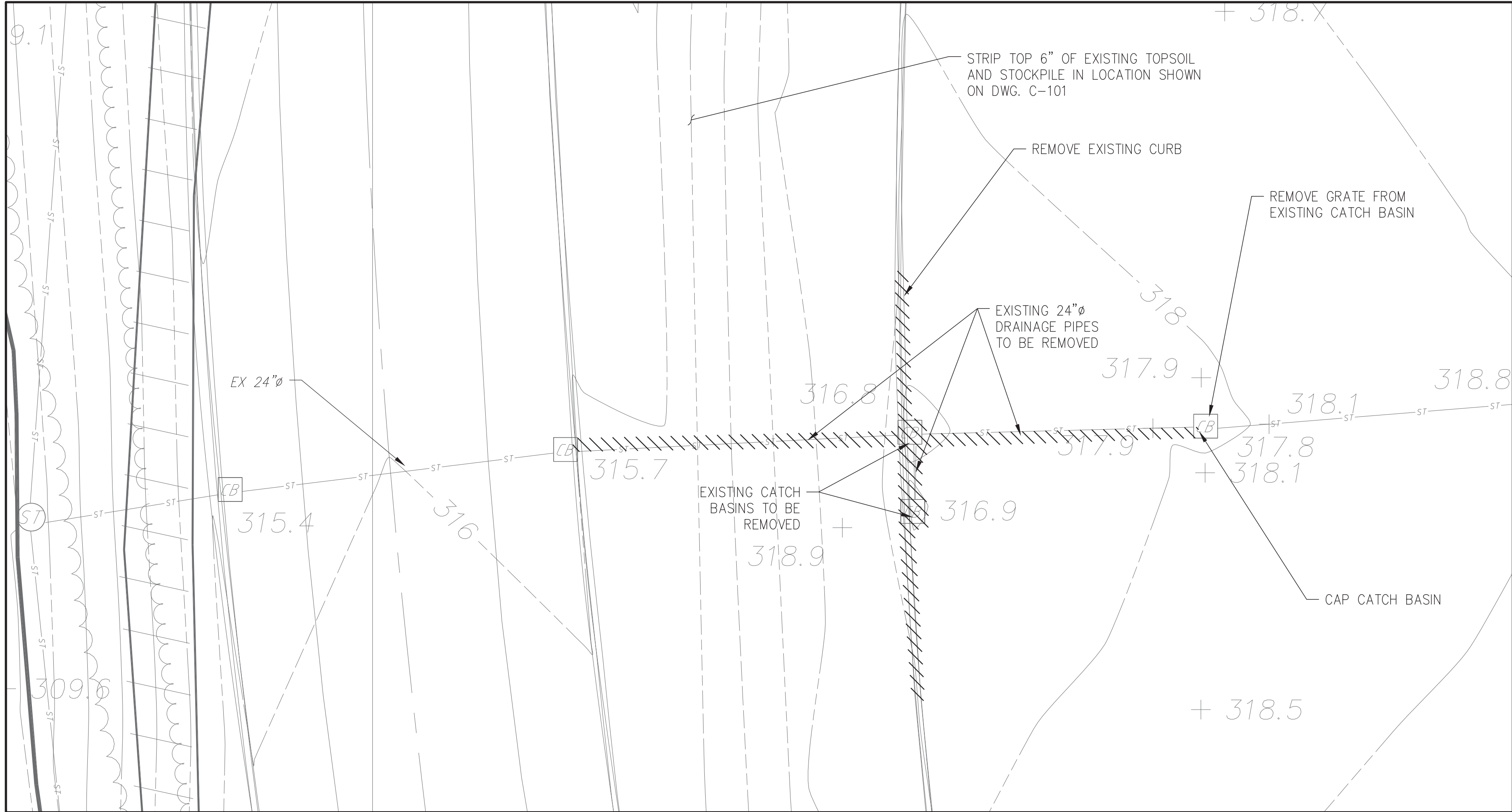
N3 PLAN SCALE: 1" = 10'-0"
