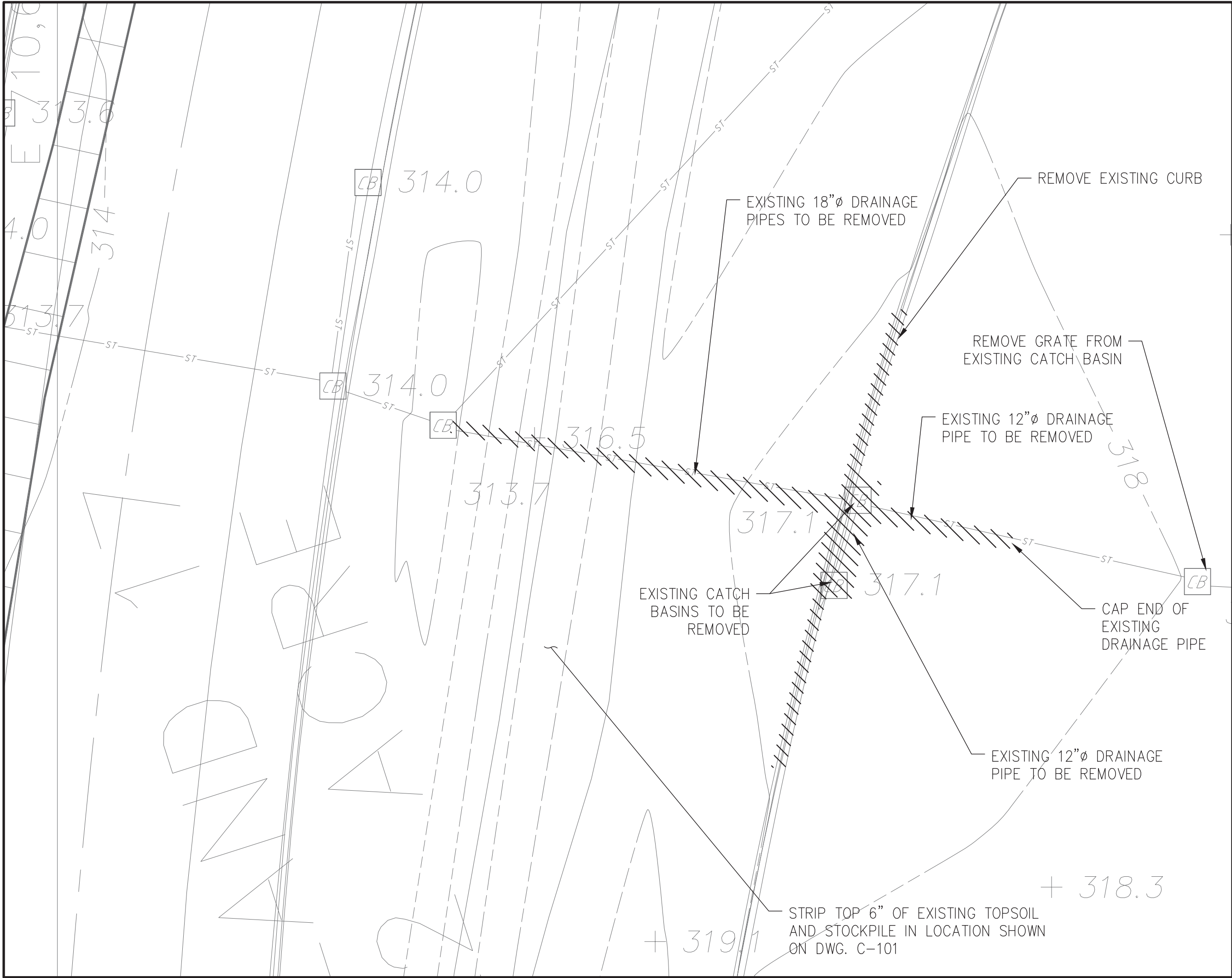
N2 PLAN SCALE: 1" = 10'-0"
