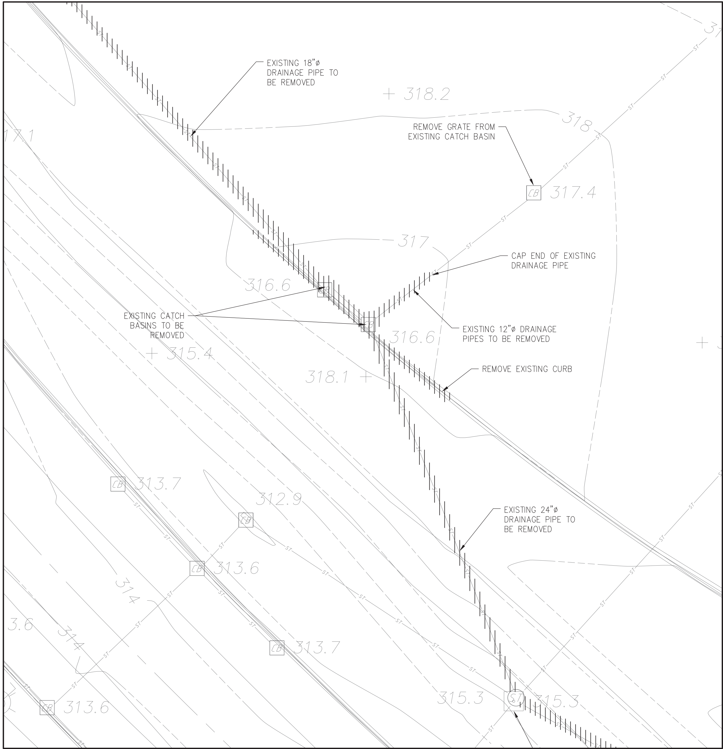
S2 PLAN SCALE: 1" = 10'-0"
