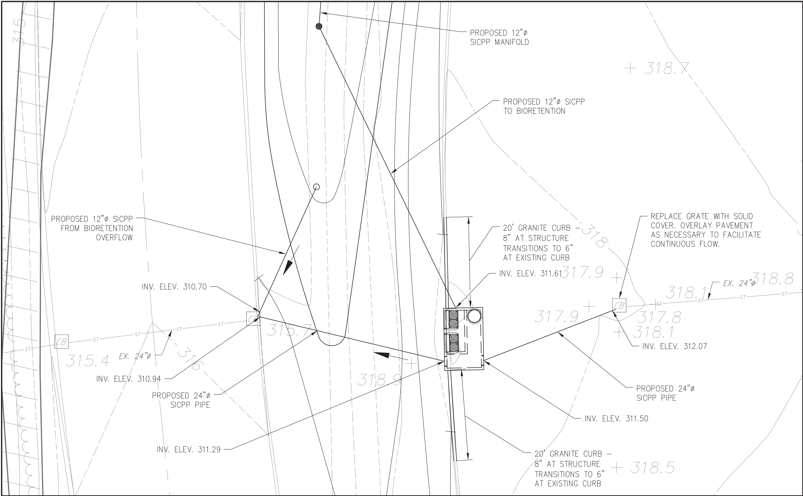
N3 PLAN SCALE: 1" = 10'-0"
