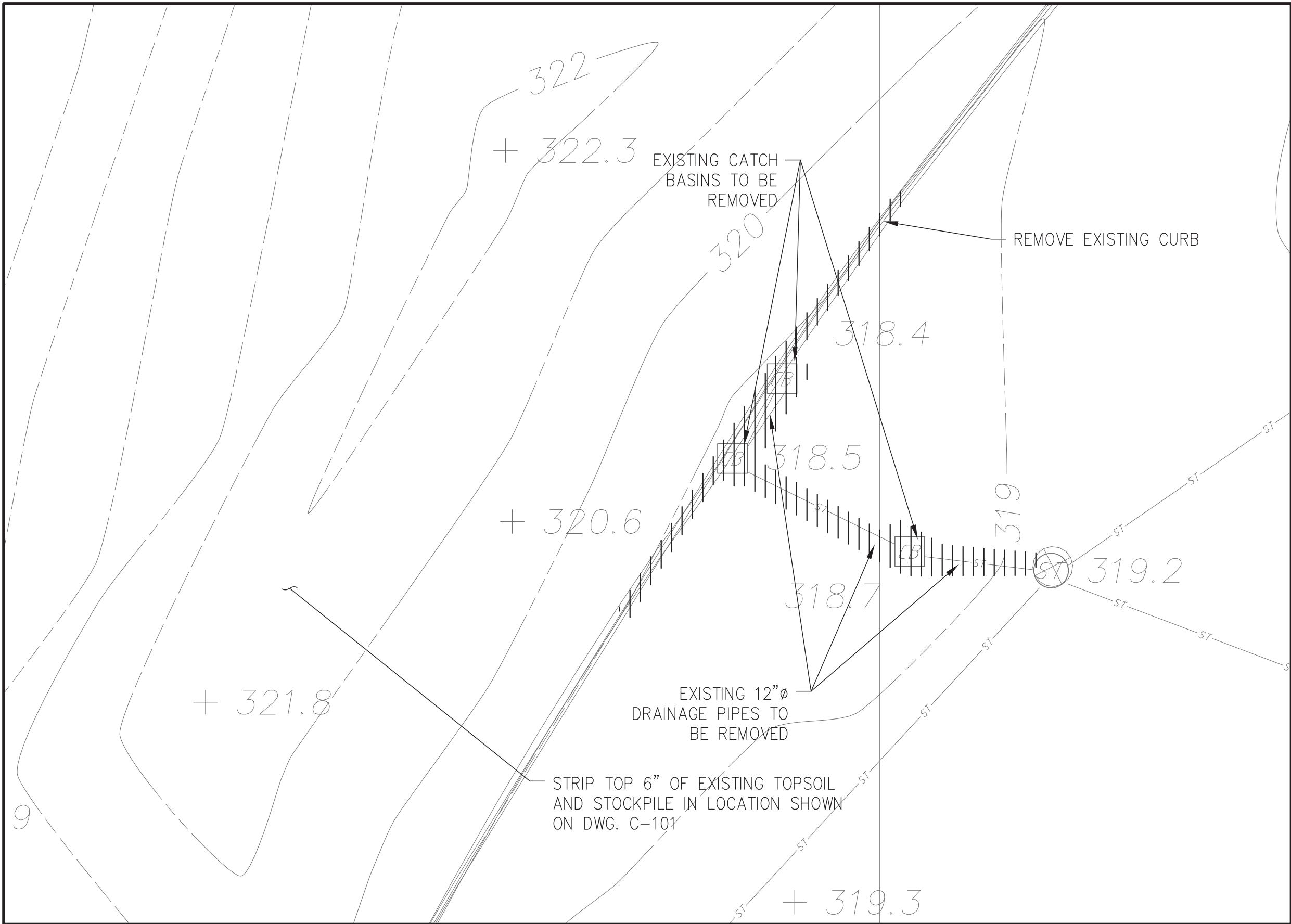
N1 PLAN SCALE: 1" = 10'-0"
